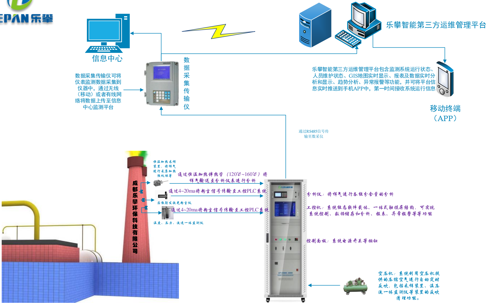
乐攀环保废气在线监测系统组织流程图
